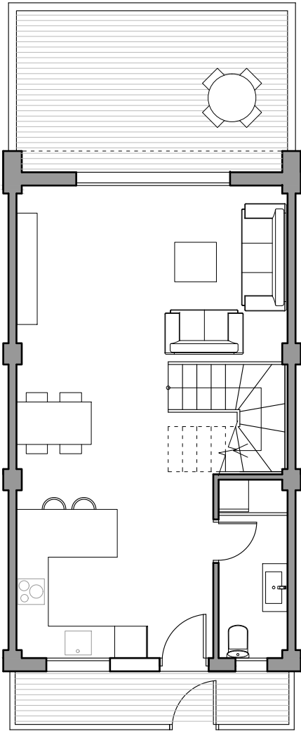
PLANTA BAJA
